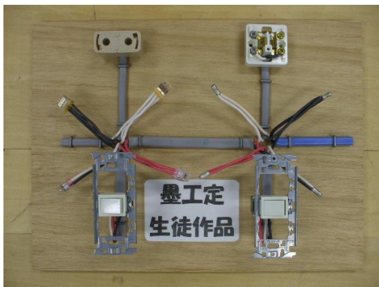
電気工事作品①
