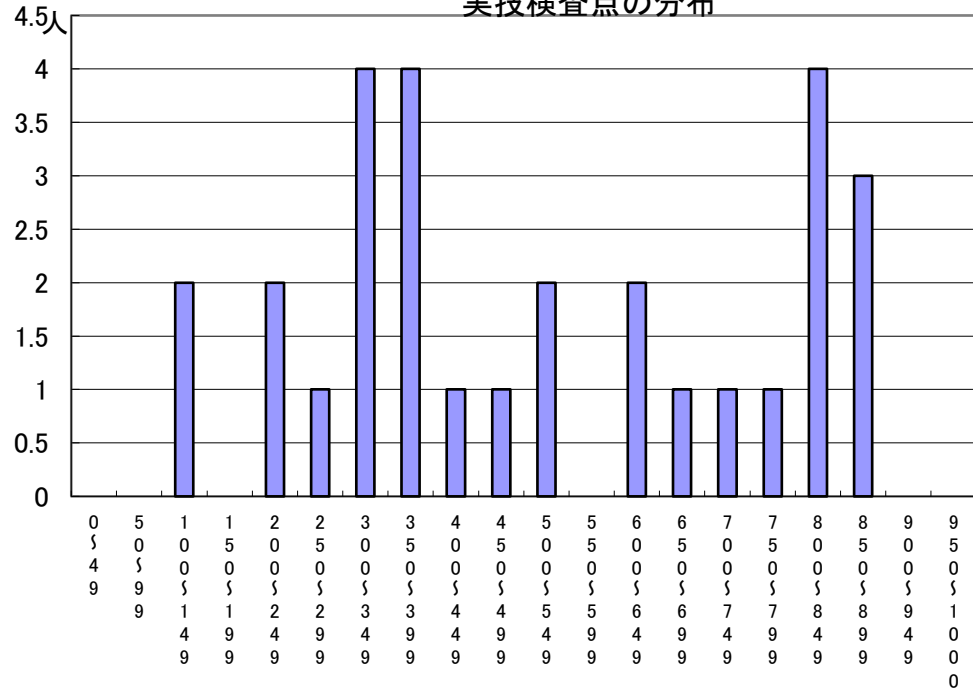
実技検査点の分布
