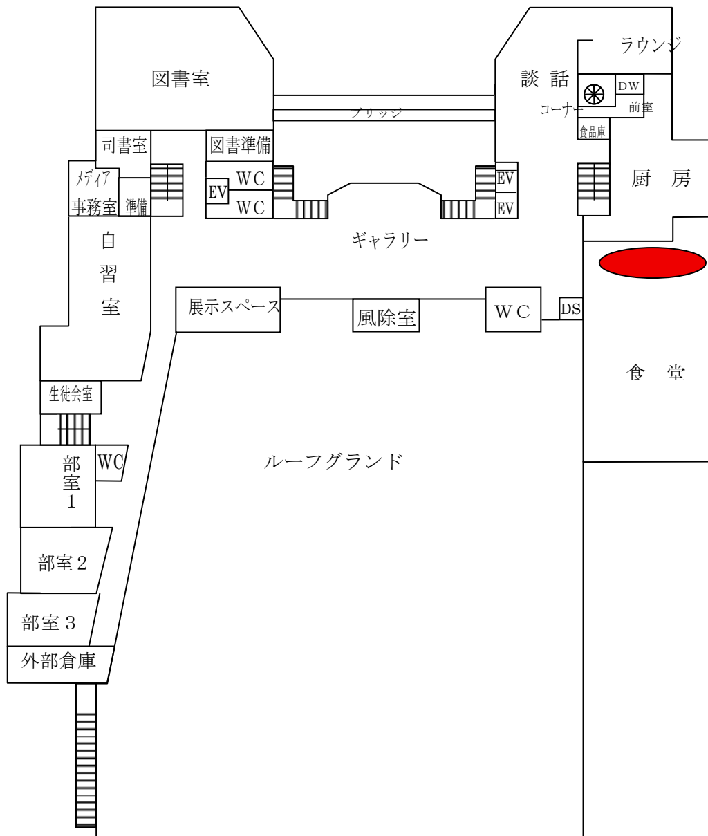
2階平面図
