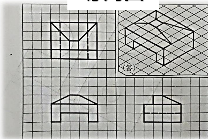
等角図
