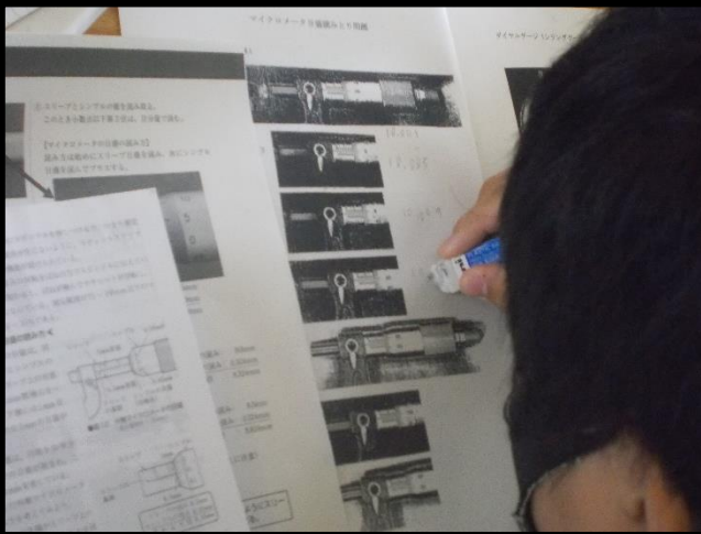
【技能検定 機械検査 3 級】 0 点合わせの調節を行っています。
