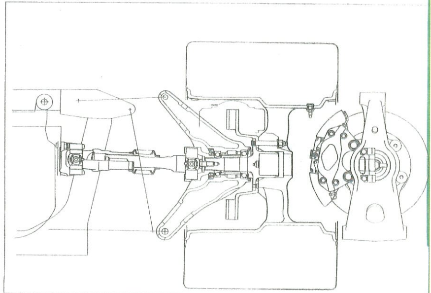
R382 リヤ・アクスル図
