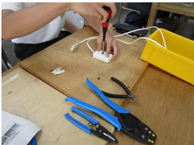
テーブルタップ（延長コード）の製作
