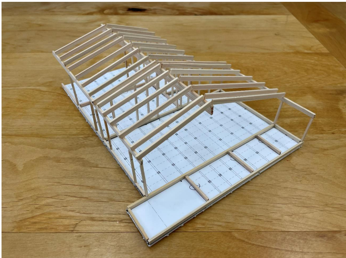
写真2 構造模型の写真
