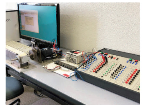
シーケンス制御実習装置
